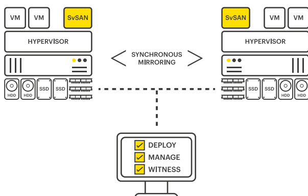
Abb. 1: Eine typische SvSAN-Konfiguration mit zwei Knoten
